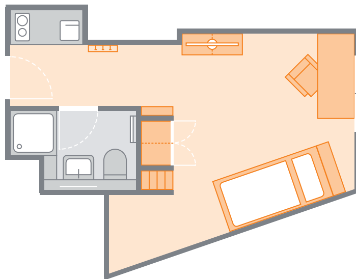
5. Grundrisstyp E
